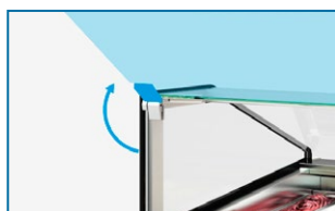
Vitrage frontal avec ressort à gaz.
